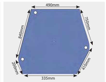
D6619 Door Glass Right Hand & Left Hand 600
