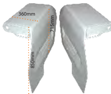
63333 Mudguard 135 165 715mm Pair
